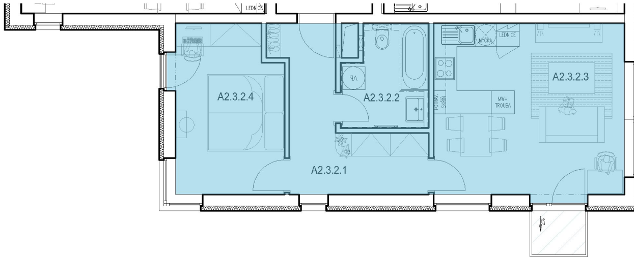
schéma podlaží
