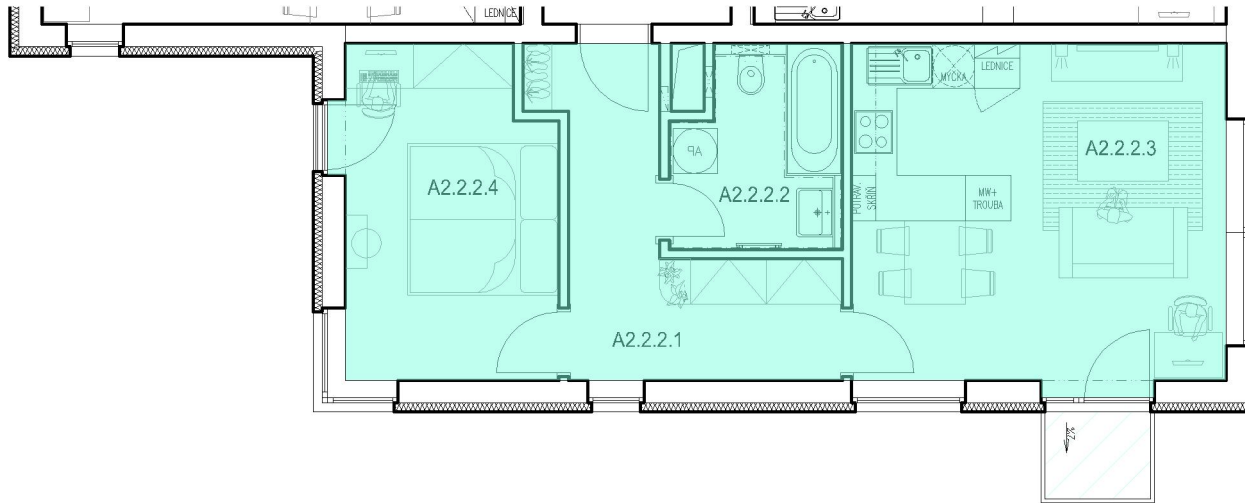
schéma podlaží
