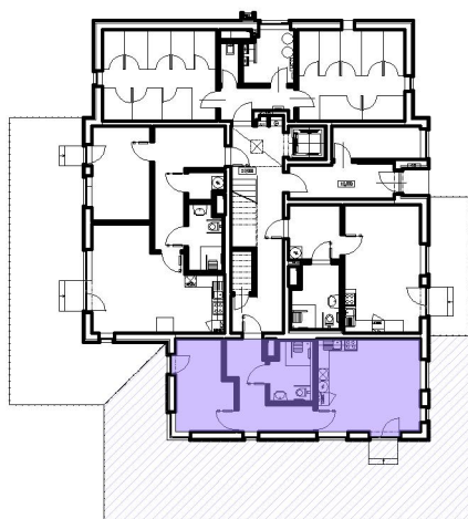
schéma podlaží
