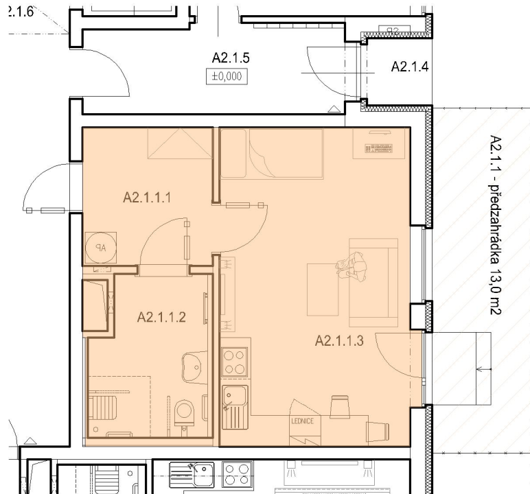
schéma bytu
