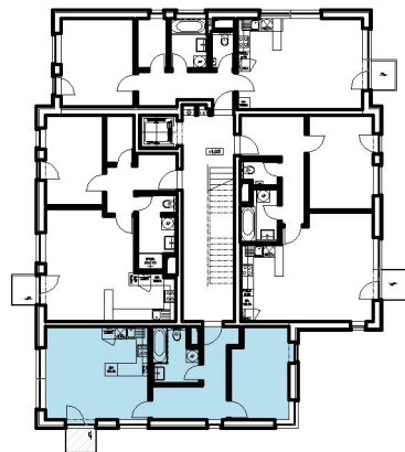
schéma podlaží
