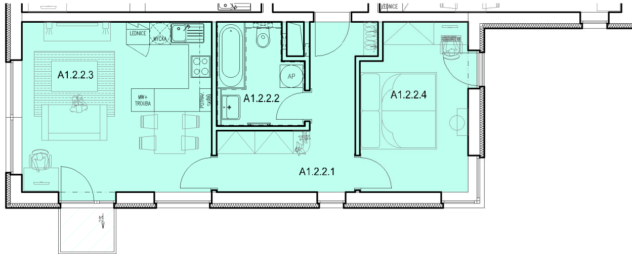
schéma podlaží
