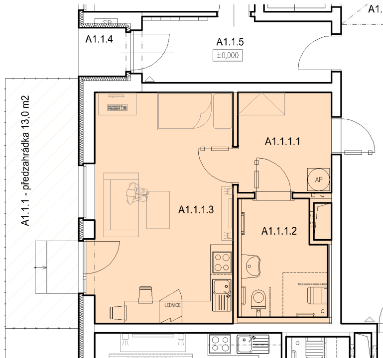
schéma bytu
